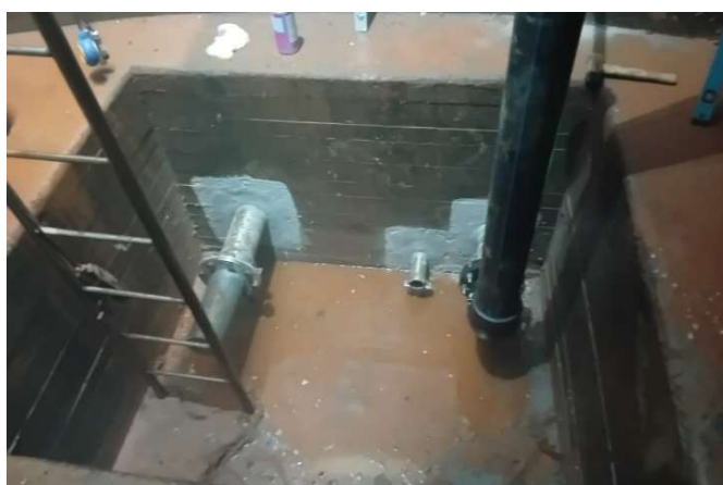
Trubní vývody v prostoru sacího koše v ak. nádrži
